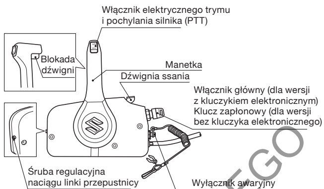
MANETKA ZDALNEGO STEROWANIA
